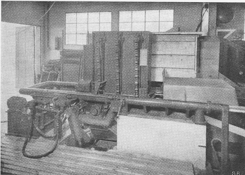
Bild 3 (links). Spanmaschine. Die auf Maschinenlänge abgeschrittenen Rundhölzer oder Holzteile werden oben eingeführt, durch die Ketten gefasst und dem Fräser zugeführt, dessen vorderes Lager sichtbar ist. Die Späne fallen in eine Grube, von der sie ein Elevator dem Sichter zuführt.
