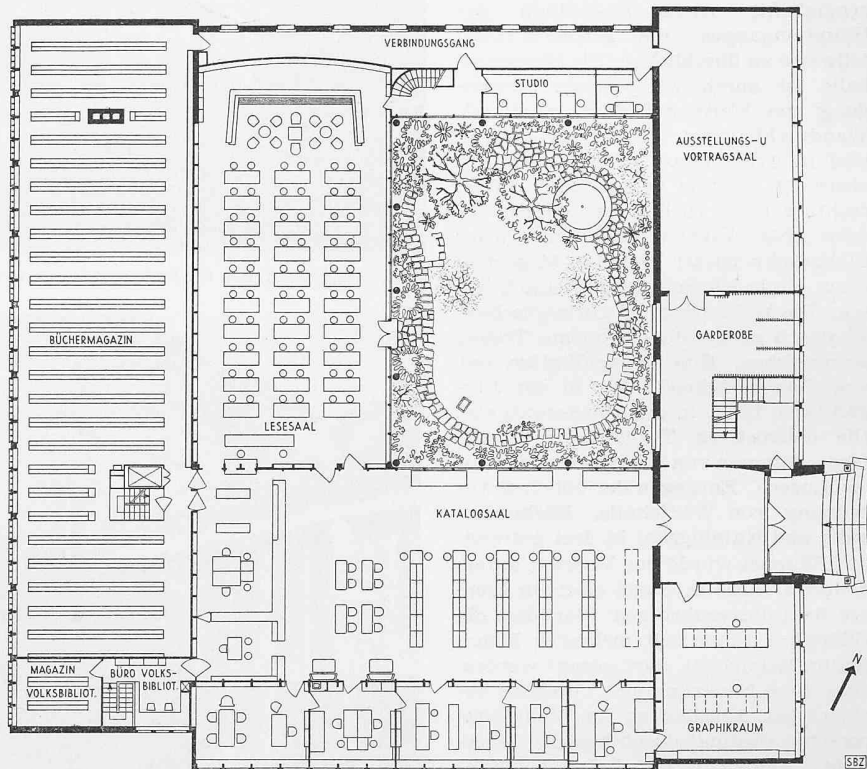
Oben Erdgeschoss, unten Keller, links Hirschmatt-, rechts Sempacherstrasse
