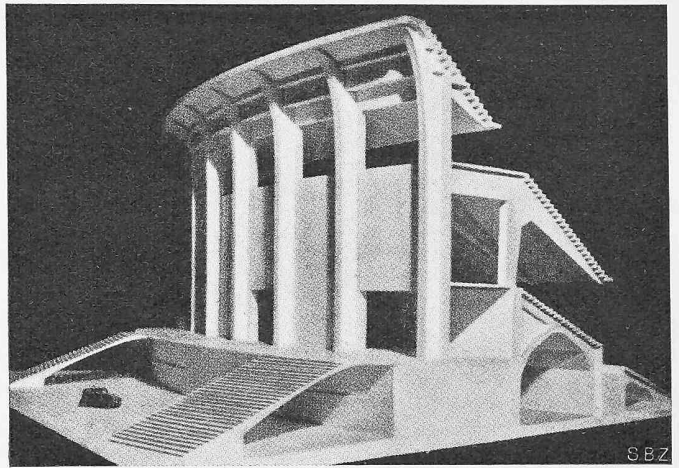
Bild 24. Projektmodell für ein Stadion in Rom. Dreistöckige Anlage, Zugang zum Ringbalkon über Tangentialtreppe, 104 000 bis 165 000 Plätze. Ing. P. L. NERVI und C. VALLE [1].
