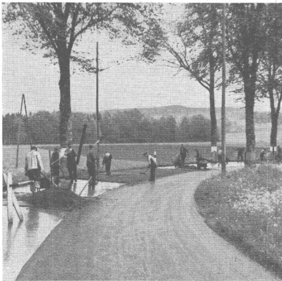
Einbau eines CARPAVE-Teppichs
