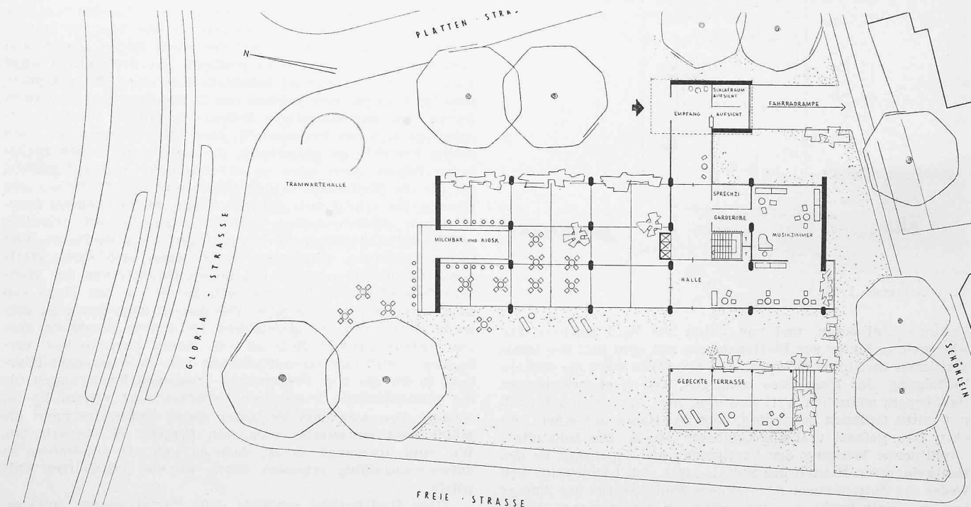
Erdgeschoss 1:600
