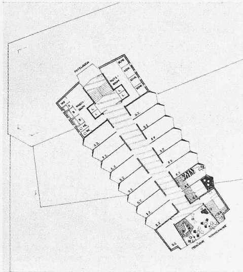
Normalgeschoss 1:600
