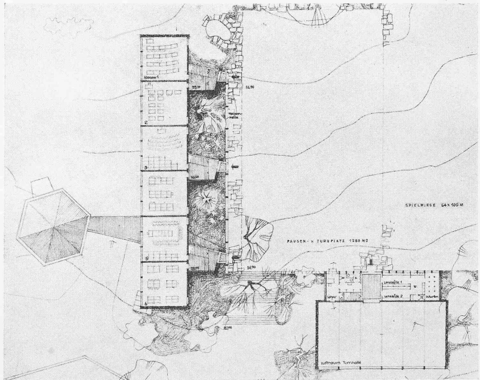
Obergeschoss, Masstab 1:700
