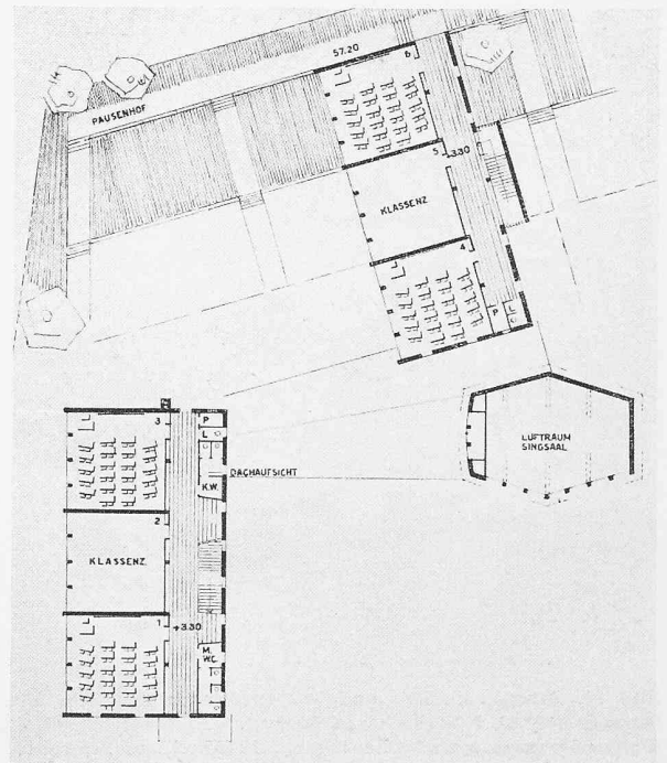
Obergeschoss
