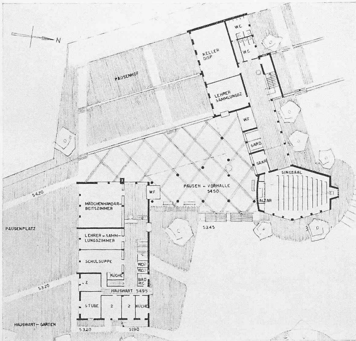
Erdgeschoss 1:700
