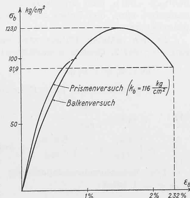
Bild 3. Spannungs-Stauchungsdiagramm
