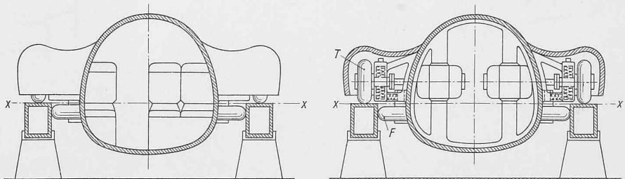
Bilder 5 und 6. Querschnitt des vorgeschlagenen Fahrzeuges durch den Passagier- bzw. durch den Motorraum
