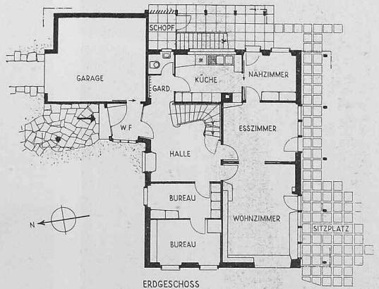
Erdgeschossgrundriss 1:300
