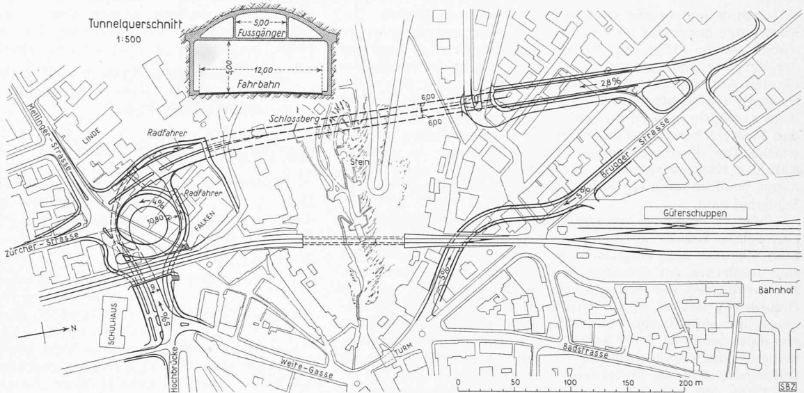
Bild 17. Bereinigter Vorschlag des Kantons und der Badener Behörden. Hauptmerkmale: die Strasse Basel-Zürich wird à niveau durchgeführt. Zur Gewinnung der Weglängen wird eine Wendel angeordnet. Die Radfahrer erhalten eigene Wege
