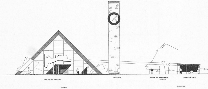
Südsansicht, Masstab 1 : 500
