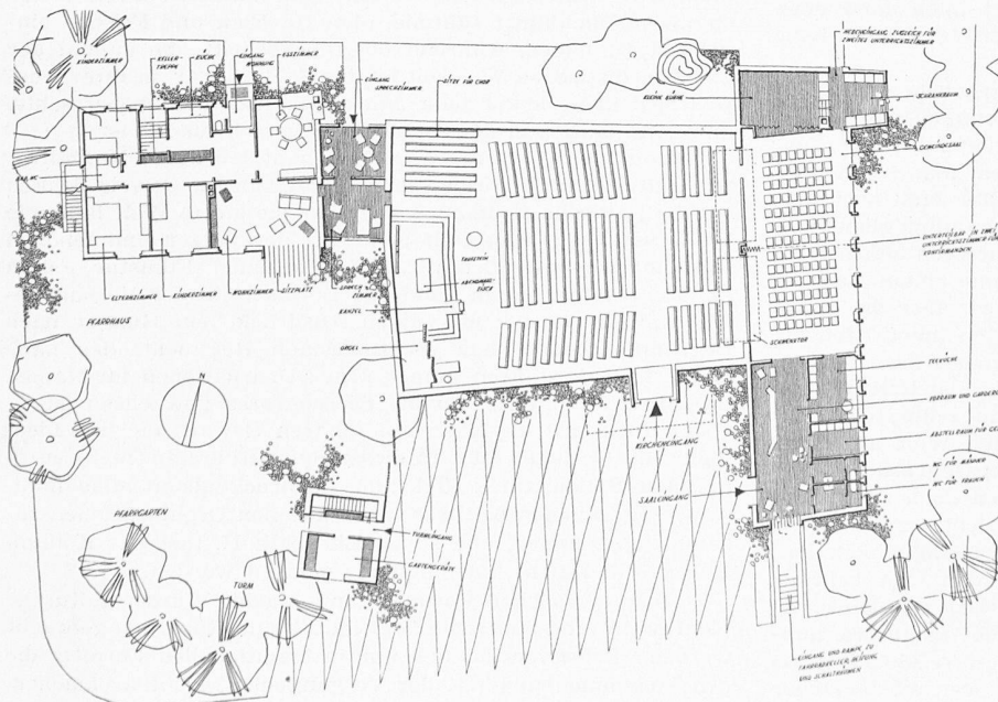
Grundriss, Masstab 1 : 500
