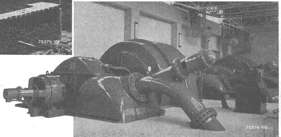
Aussenansicht und Maschinensaal des Wasserkraftwerkes «Juan Carosio», Moyopampa (Peru)
