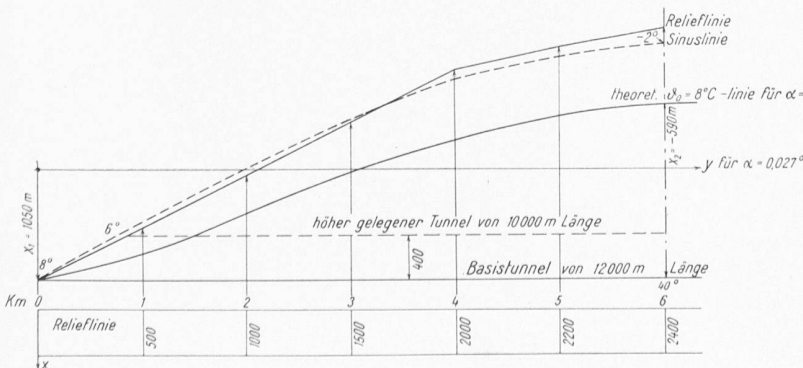
Bild 4. Schematisches Beispiel für h/l = 1/10
