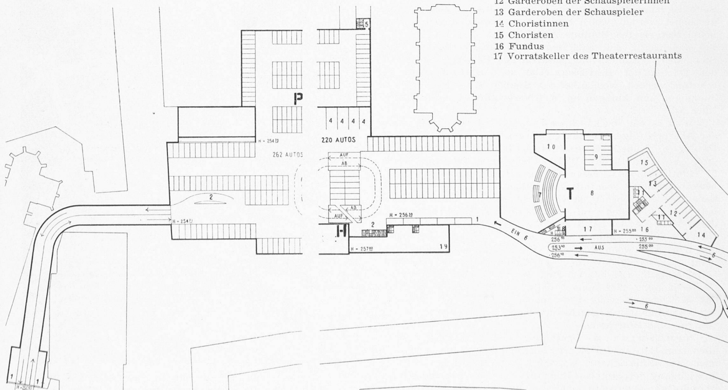
2. Parkingkeller, Masstab 1:1500
