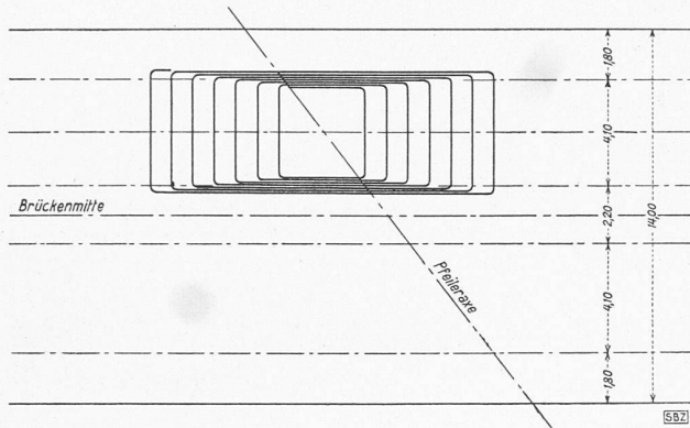
Bild 6. Projekt Nr. 10c, Spannbetonssystem Dr. Heilig und Besemer, Grundriss 1:300, mit schematischer Andeutung des Verlaufs der Spannarmierung für gleichzeitige Längs- und Quervorspannung. Verfasser Ing. H. AEBERHARD, Thun. Unternehmer F. TRACHSEL, Frauenfeld, H. ZÜST, Wattwil. Kosten rd. 1 000 000 Fr.
