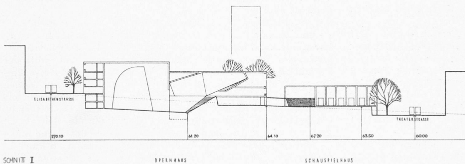
SCHNITT I
