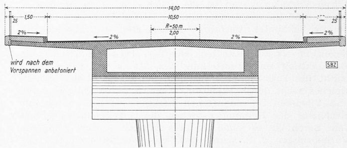
Bild 8. Querschnitt 1:150
