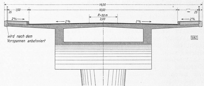
Bild 8. Querschnitt 1:150
