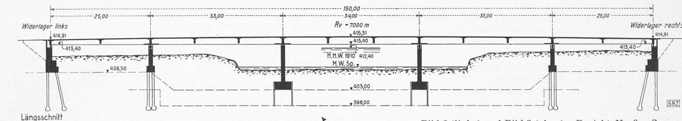
Bild 2 (links) und Bild 3 (oben). Projekt Nr. 3c, Spannbetonsystem BBRV, Grundriss und Längsschnitt 1:900. Verfasser Ingenieure E. SCHUBIGER, Zürich, WEDER und PRIM, St. Gallen. Unternehmer LOCHER & CIE., Zürich, H. STUTZ AG., Hatzwil. Kosten 844 833 Fr. Zur Ausführung bestimmt.
