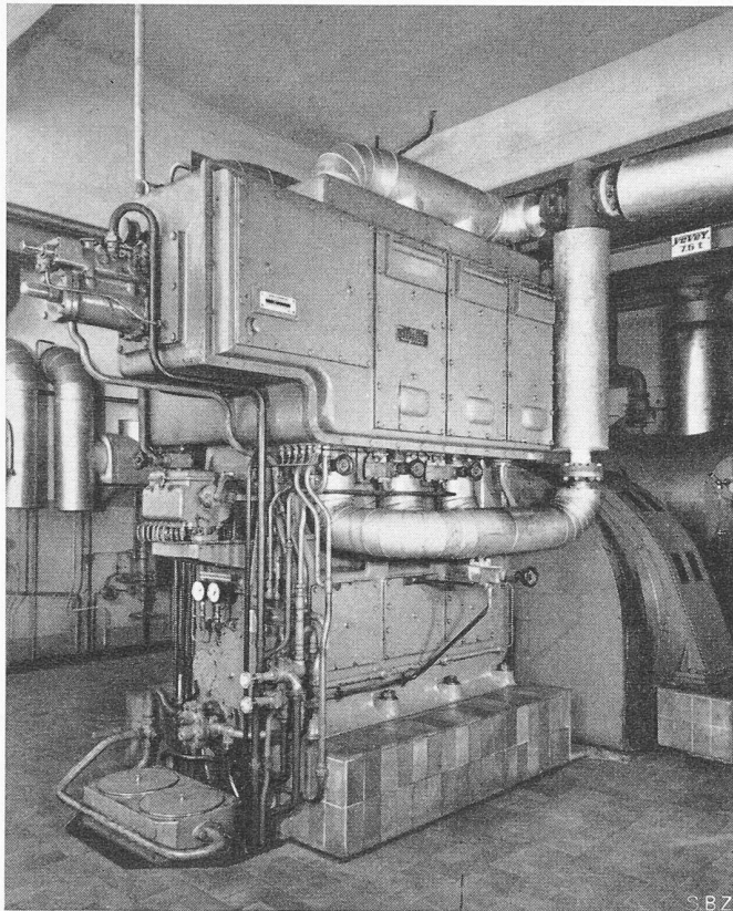
Bild 5. Dreizylindermaschine 1150 PS, Einlasseite
