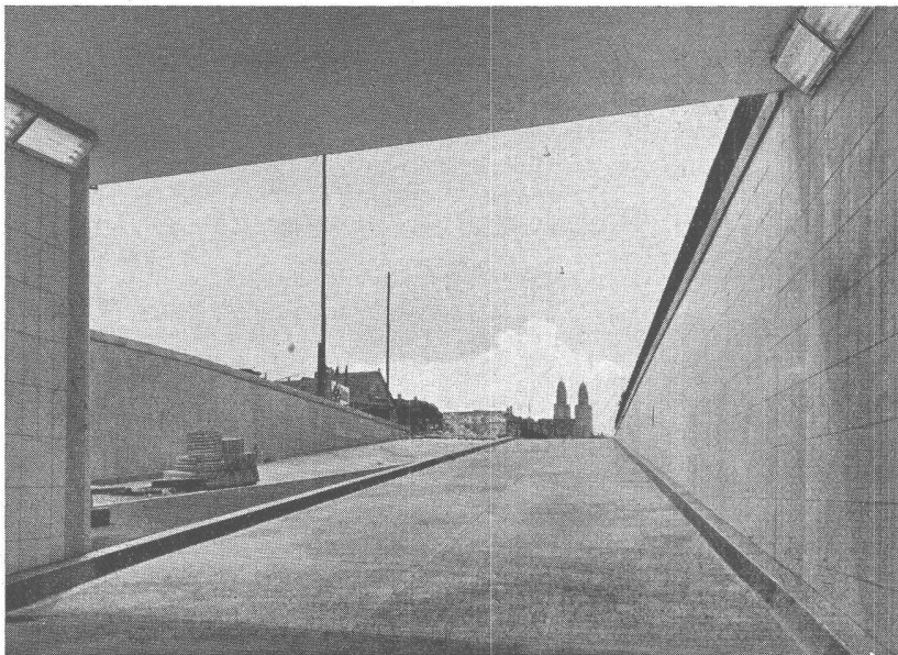
Unterführung Bahnhofquai Zürich, 1. Etappe Isolierung des Troges gegen Grundwasser und Deckenisolierung ca. 2000 m 2 Bauleitung: Tiefbauamt der Stadt Zürich Eisenbetonarbeiten: H. Eichenberger, Ingenieurbüro, Zürich
