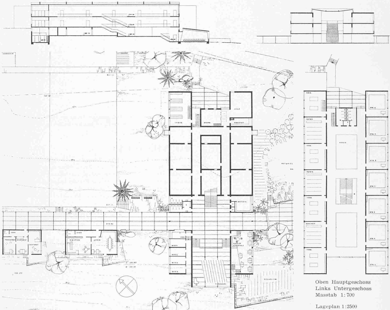
Nicht prämiertes Projekt von Dipl. Arch. H. VON MEYENBURG, Zürich.
