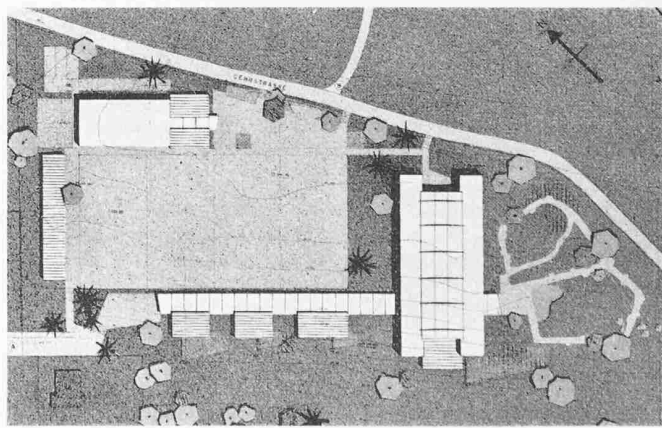
Oben Hauptgeschoss Links Untergeschoss Masstab 1:700 Lageplan 1:2500
