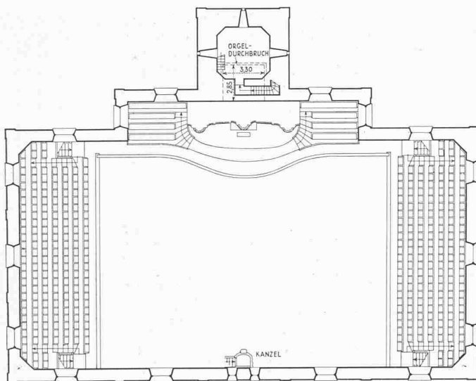
Emporengeschoss, Masstab 1:400
