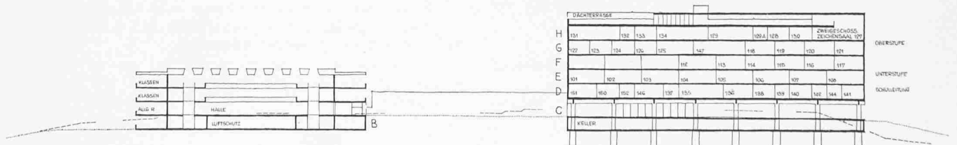
Längsschnitt Ost-West
