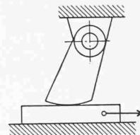
Bild 1. Bewegungssperre durch Daumen für Rechtsbewegung
