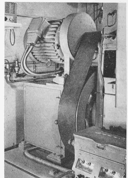
Bild 5. Schwenkmotor von 10 PS als Antrieb für einen Höchstdruckkompressor
