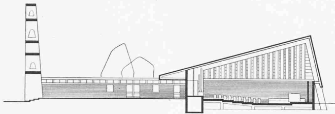
SCHNITT GLOCKENSTUHL - HOF - KIRCHE/EINGANG PFARRER / DETAIL FENSTERLAMELLEN SIEHE IM ERLÄUTERUNGSBERICHT
