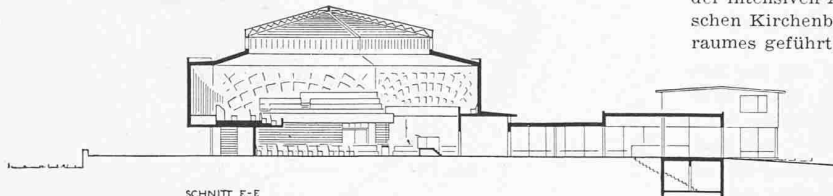
SCHNITT E-E
