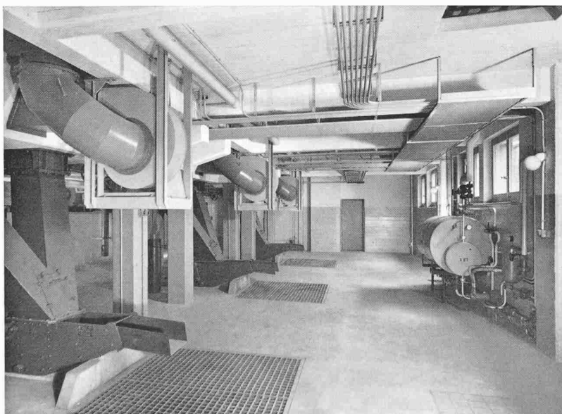
Unterwindventilatoren und Halbbrassentschläcker im Geschoss B des Kesselhauses, rechts Brennölversorgungsinstallation
