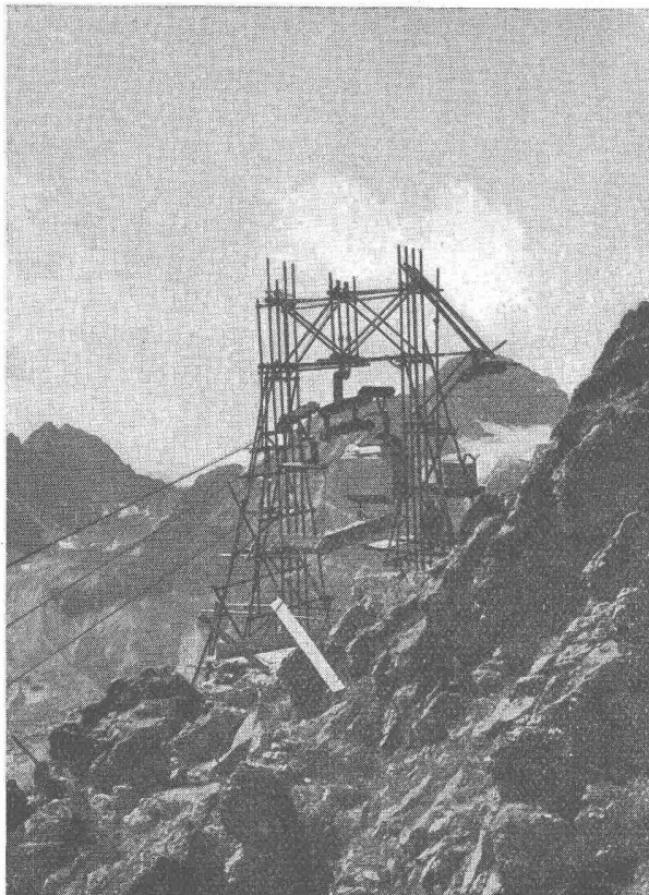
Provisorischer Portalmast für Seilbahn Corviglia-Piz Nair 2800 m ü.M. August 1953
