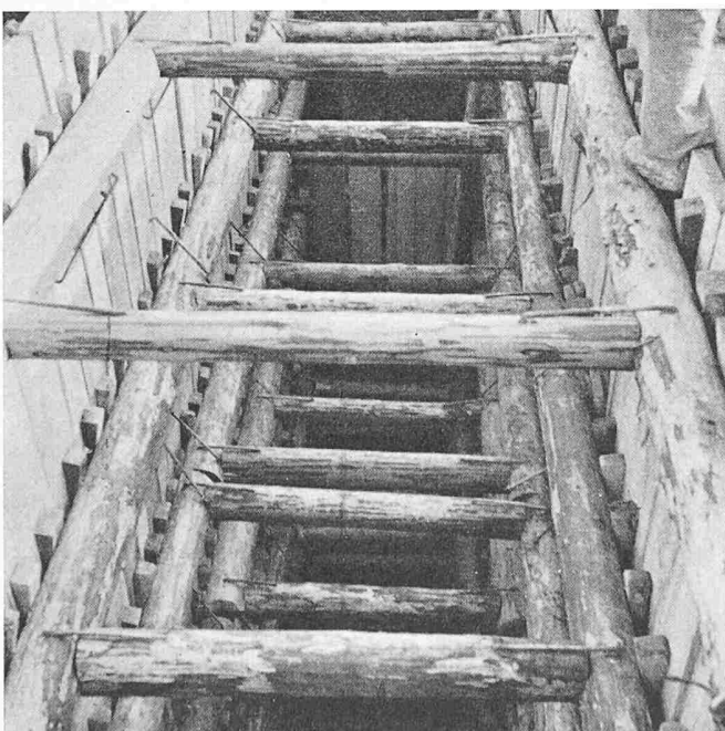
Die Spriessung im ausgehobenen Sporren in Axe 8; Tiefe 12 m
