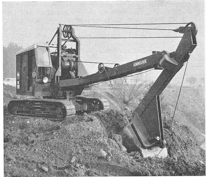
P & H-Raupebagger mit Tieflöffelausrüstung und Kübel von 600 l Inhalt
