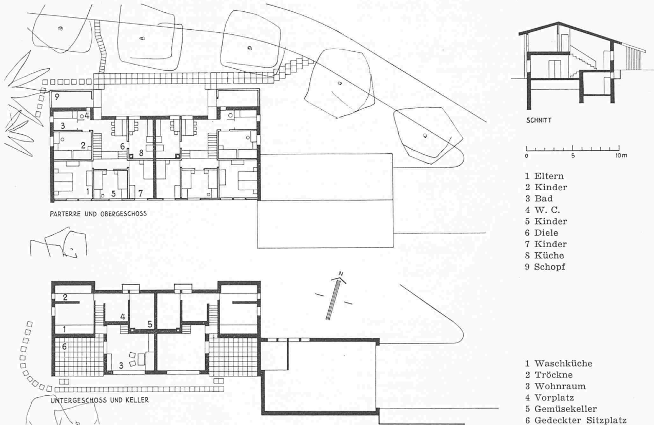
Doppelfamilienhaus für Heizer und Chauffeur, 1:400
