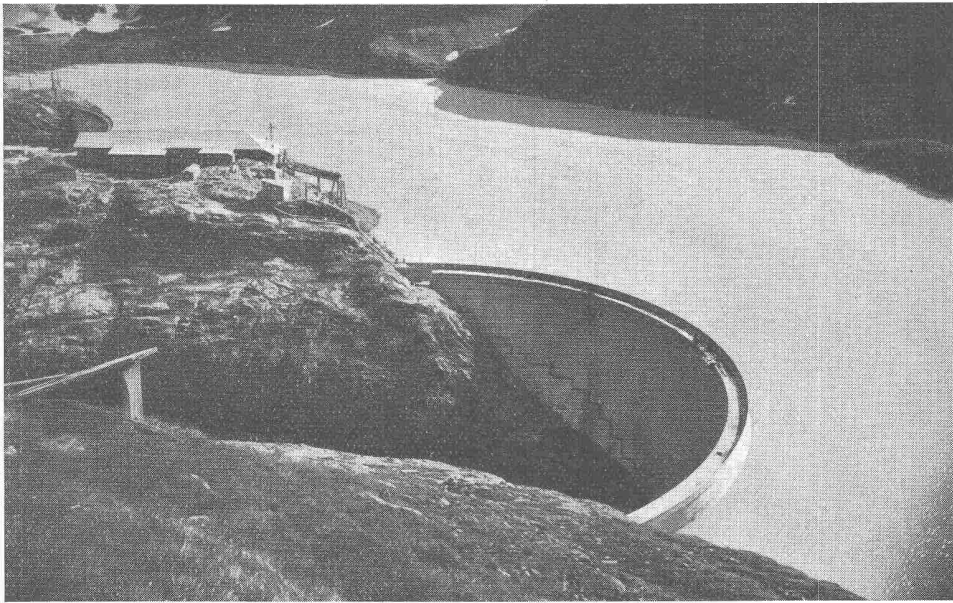
Möllsperr und im Hintergrund links Margaritzensperre, Tauernkraftwerke Kaprun-Salzburg beide Sperren erbaut in FRIOPLAST-Beton
