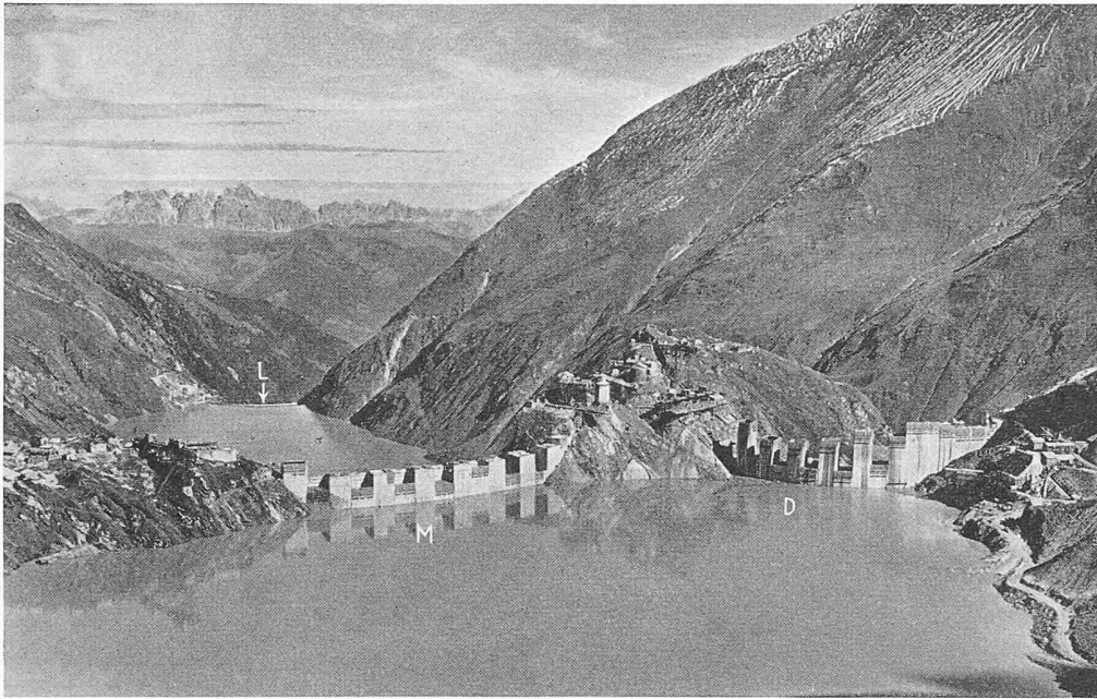
Bild 4. Speicher Mooserboden mit den Mauern Mooser (M) und Drossen (D), dazwischen die Höhenburg. Im Hintergrund die Limbergsperr (L). Bauzustand am 25. Sept. 1954
