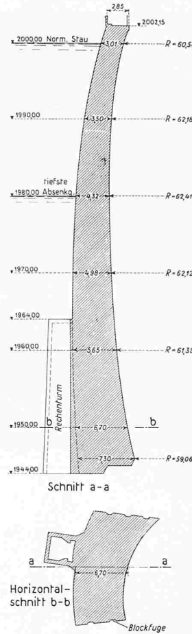
Bild 5. Möllsperre, Querschnitt 1:650
