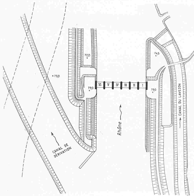
Bild 13. Kraftwerkanlage Montélimar, Lageplan 1:8000 des Stauwehres Rocheamaure
