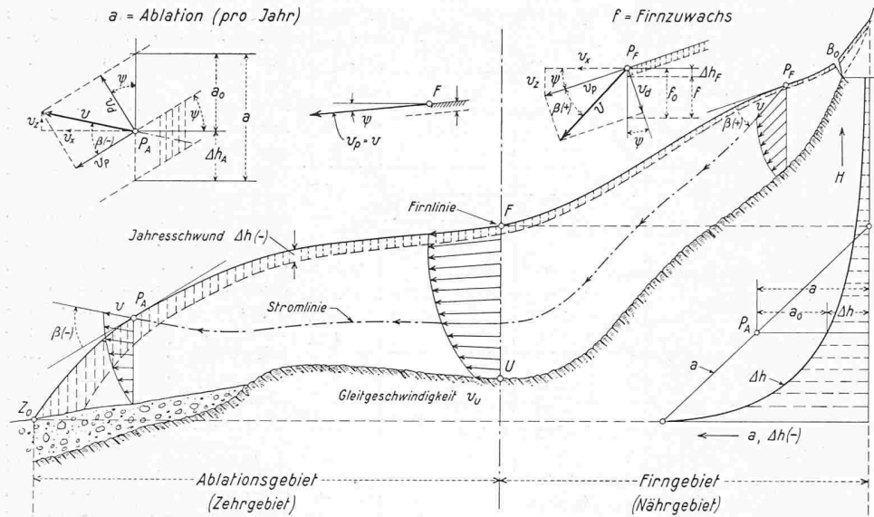
Bild 4. Beziehungen zwischen der jährlichen Höhenänderung der Gletscheroberfläche und der Fließgeschwindigkeit (Längenprofil, schematisch)
