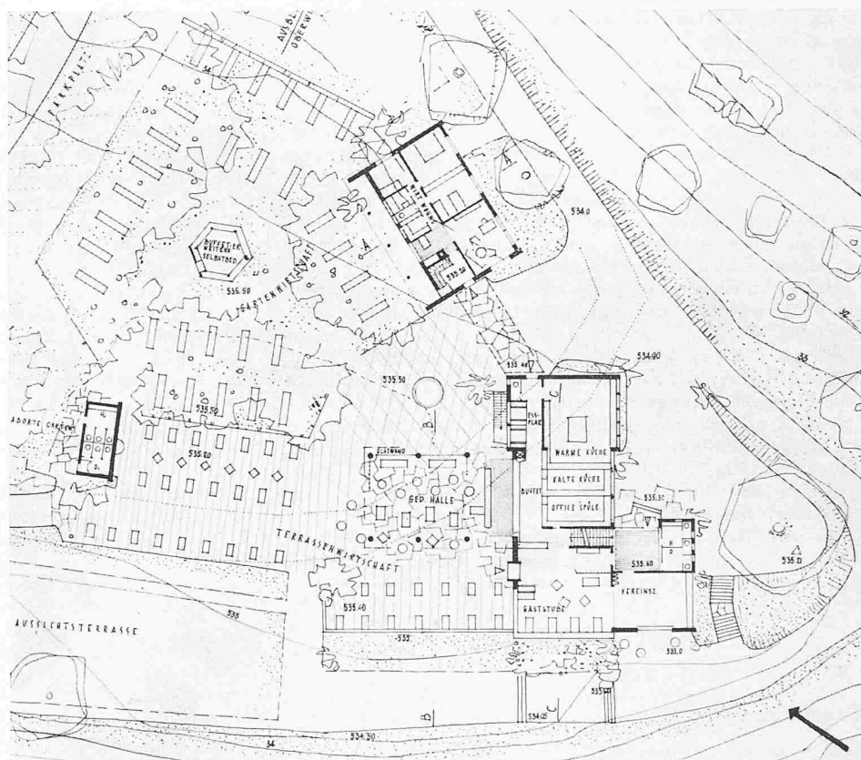
Grundriss 1:600
