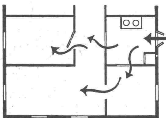
Falsch: Küchenfenster geöffnet. Ueberdruck in der Küche. Die Luftbewegung arbeitet von der Küche gegen die Wohnräume. Die Kochdämpfe dringen in die Wohnräume, auch wenn die Türen geschlossen sind.
