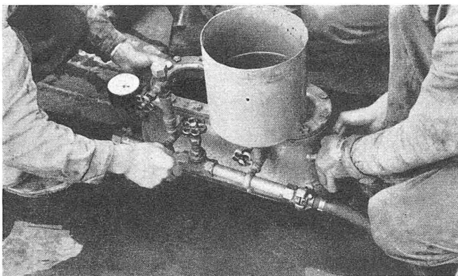
Bild 3. Prüfung der Bodenschweissnähte mit der Vakuump-Haube
