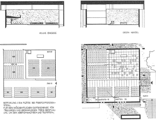
Grundriss (mit verschiedener Bestuhlung) und Schnitte Obergeschoss (Kirchenraum)
