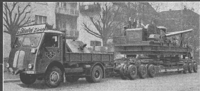
Transport eines 54 Tonnen schweren Rammenfusses auf dem 24fach bereiften Schwertransportanhänger mit dem starken Allrad-Zugwagen mit Seilwinde.
