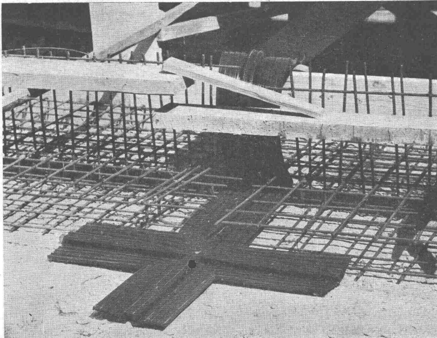
Abdichtung eines Fugenkreuzes
