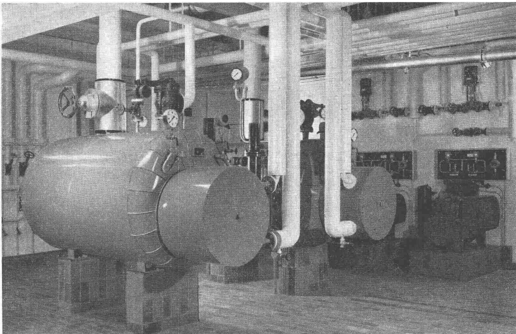
Heißwasser-Dampfumformer
