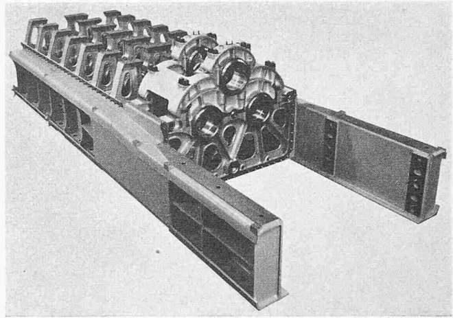
Bild 3. Geschweisstes Kurbelgehäuse
