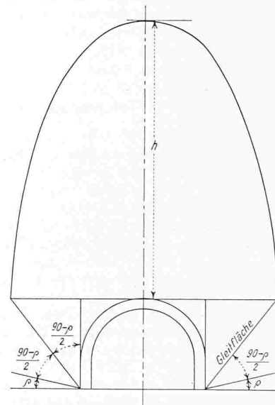
Bild 1. Druckkörper nach Kommerell
