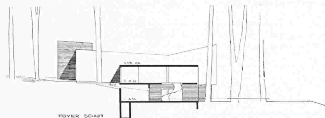
FOYER SCHNITT
