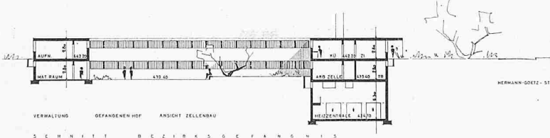
Schnitt durch das Bezirksgefängnis
