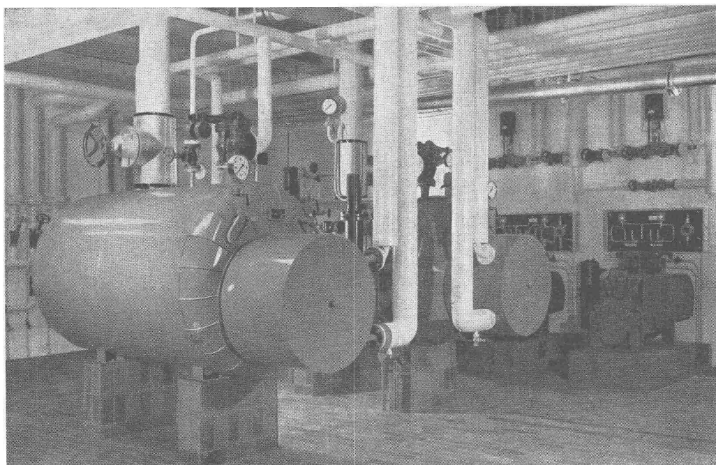
Heißwasser-Dampfumformer
