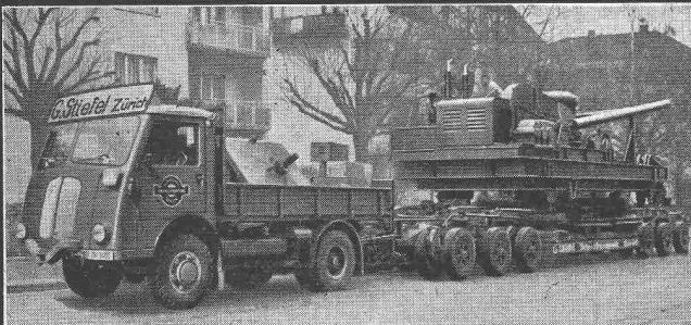
Transport eines 54 Tonnen schweren Rammenfusses auf dem 24fach bereiften Schwertransportanhänger mit dem starken Allrad-Zugwagen mit Seilwinde.
