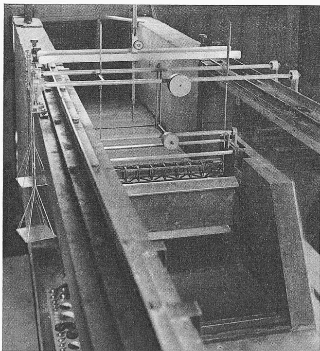
Bild 4. Versuchseinrichtung
