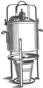
Exsiccator für Neubau-Auströcknung
