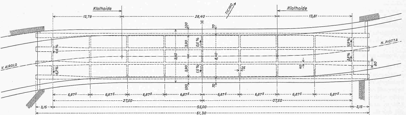
Bild 2. Grundriss 1:400
