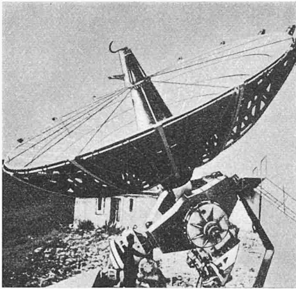
Bild 25. Sonnenglutöfen von Bouzaréah, Algier
