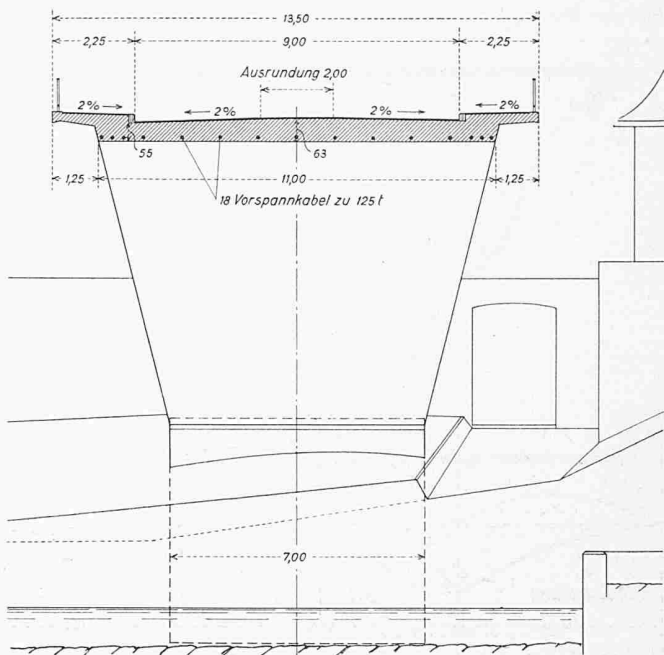
Bild 6. Querschnitt A—A, 1:200
