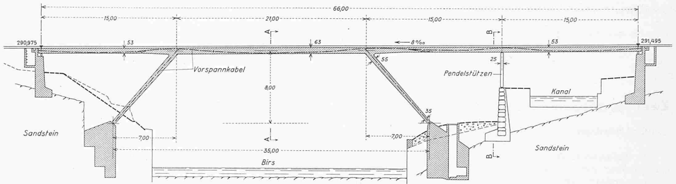
Bild 2. Birsbrücke in Dornach, Längsschnitt in Brückenaxe, 1:400
