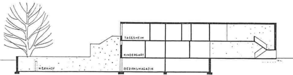
LÄNGSSCHNITT
