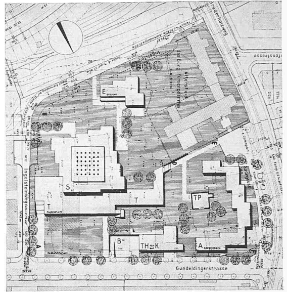
Lageplan 1:2500
