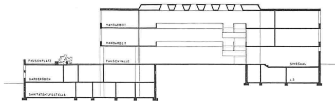
QUERSCHNITT GARDEROBEN HALLE
