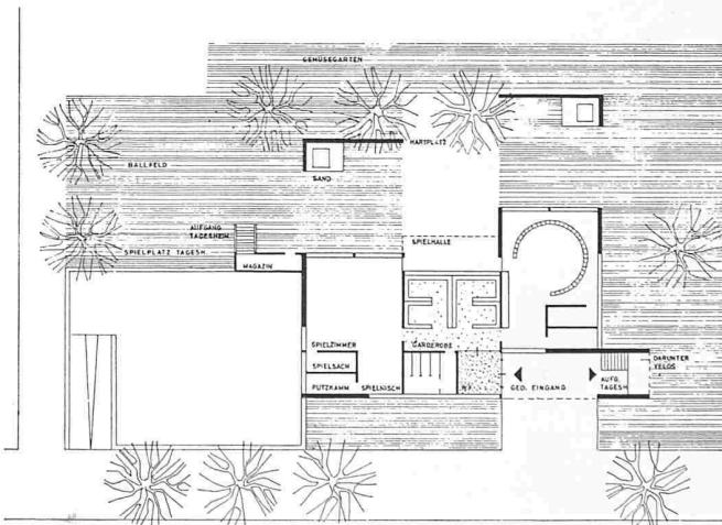
ERDGESCHOSS KINDERGARTEN
