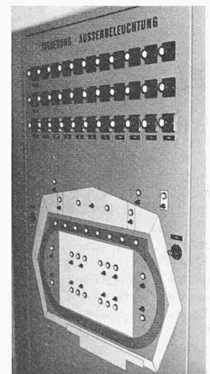
Bild 10. Schalttafel-Steuerfeld mit Blindschema
